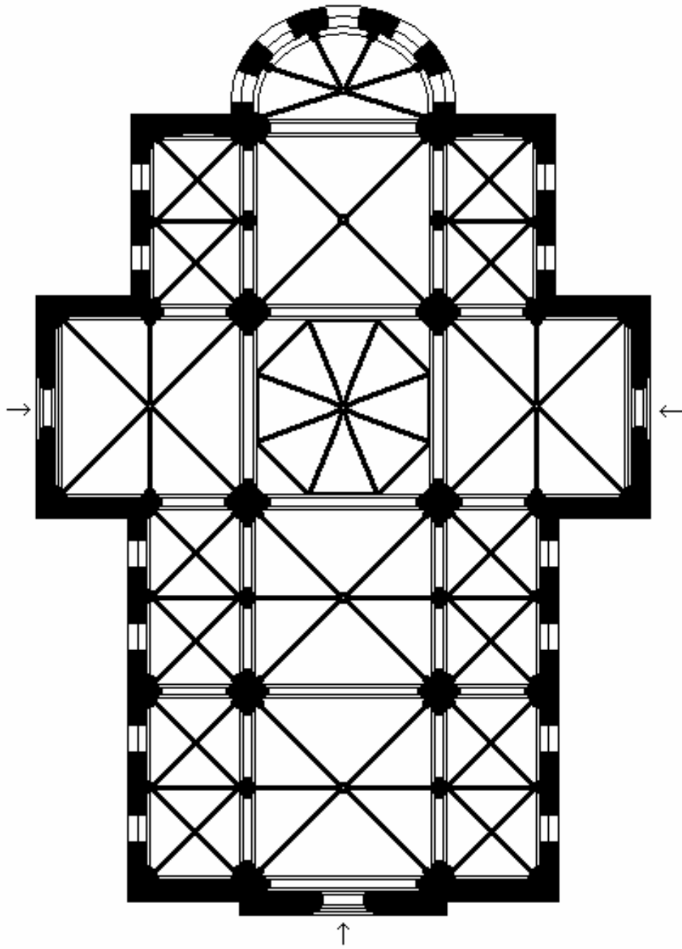
Grundriss ohne den erst später angebauten Westturm
