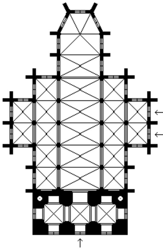
↑ Grundriss
