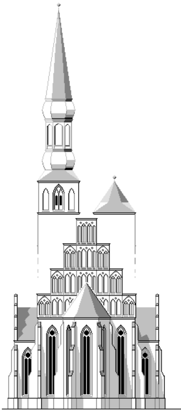
Ostansicht
